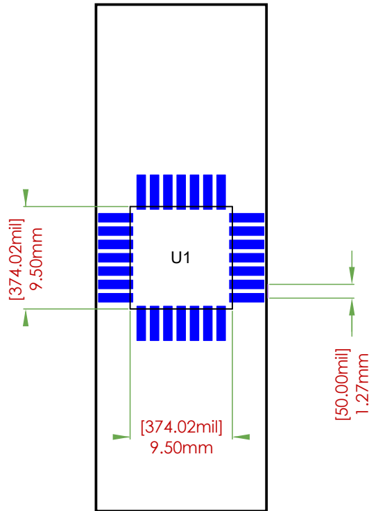
FOOTPRINT DIMENSIONS
