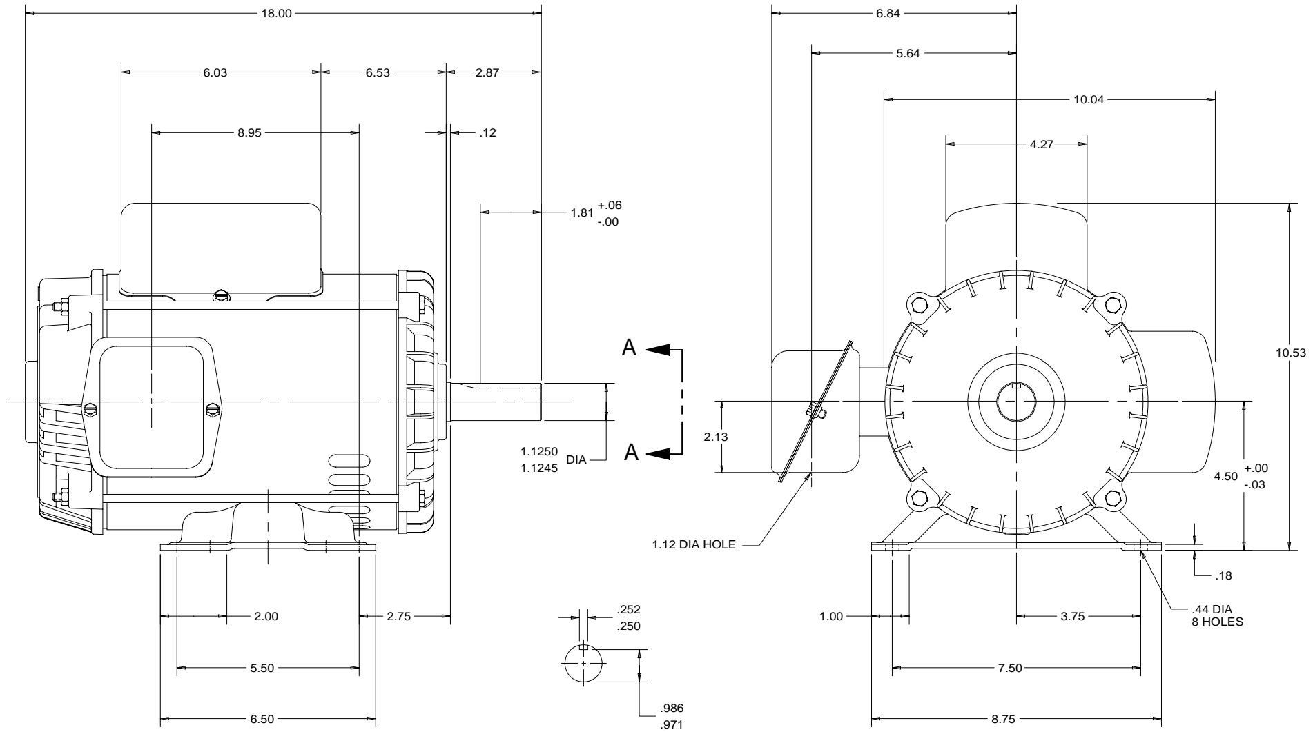
VIEW A-A
