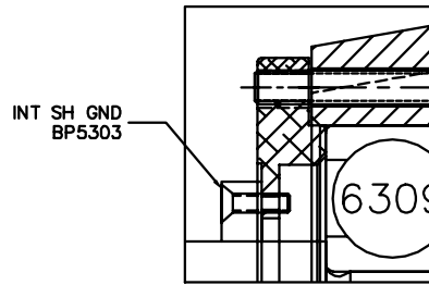
PU RETAINER DETAIL
