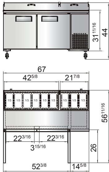
MPF8202GR
