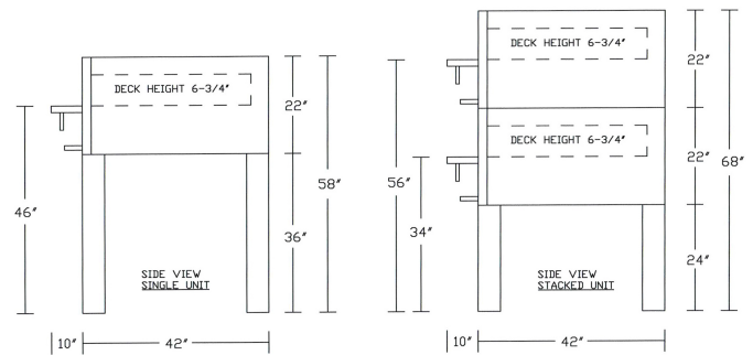
SRPO-60G | SRPO-60G-2
