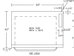
SRPO-60G | SRPO-60G-2
