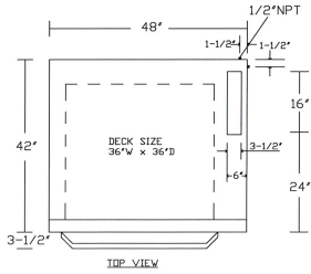
SRPO-48G | SRPO-48G-2
