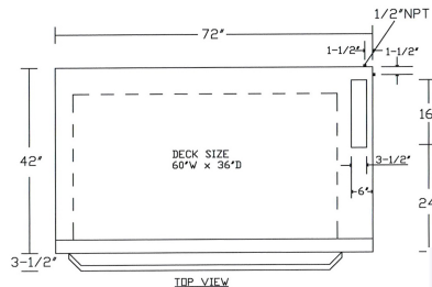
SRPO-72G | SRPO-72G-2
