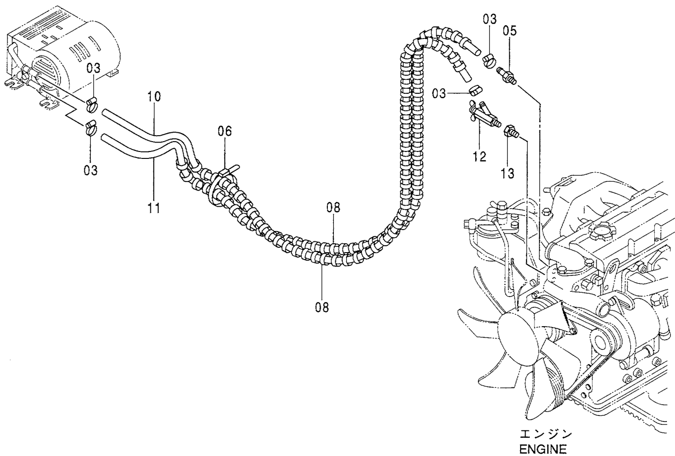
カーヒータ CAR HEATER
