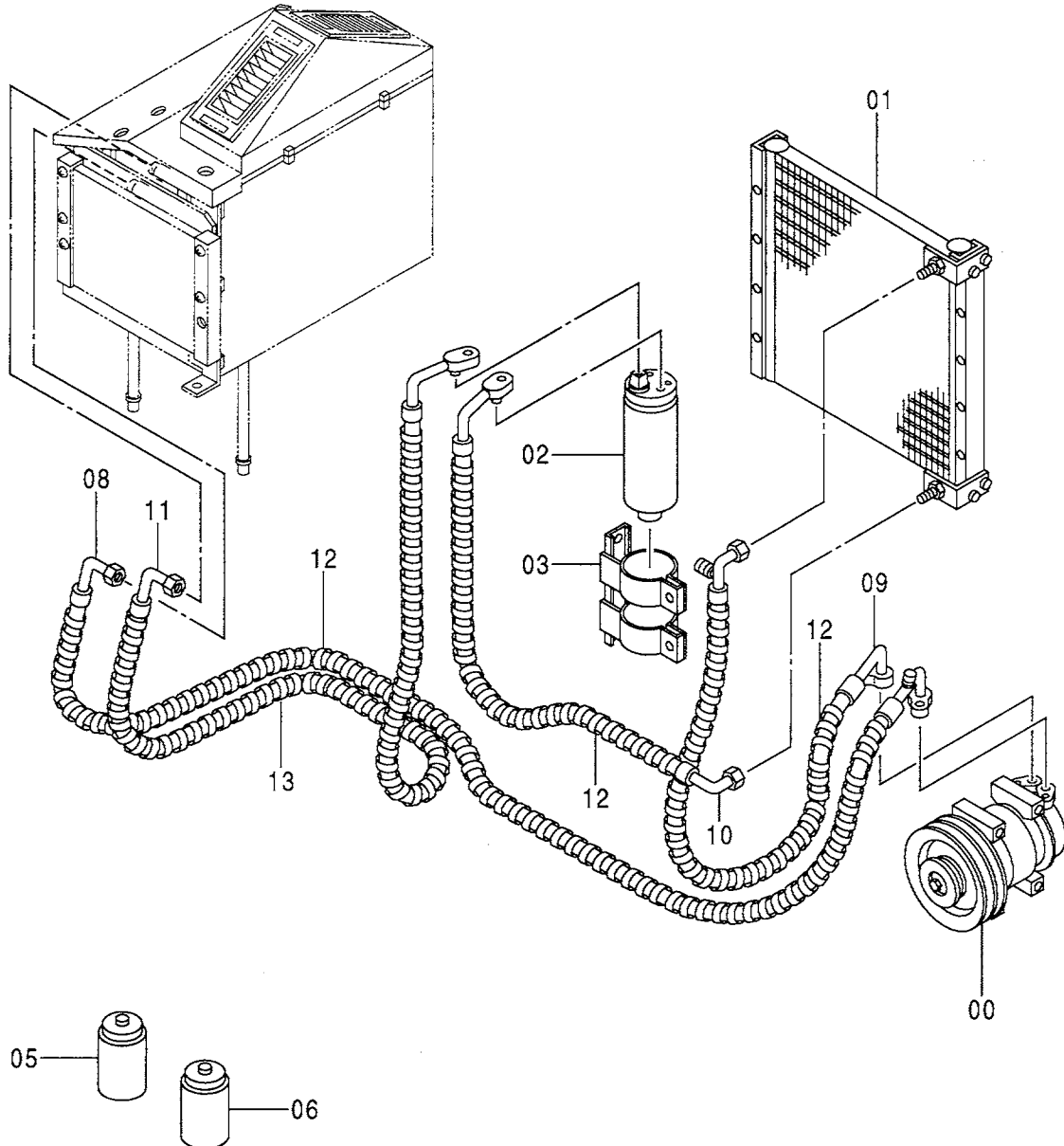
カークーラ (1) CAR COOLER (1)
