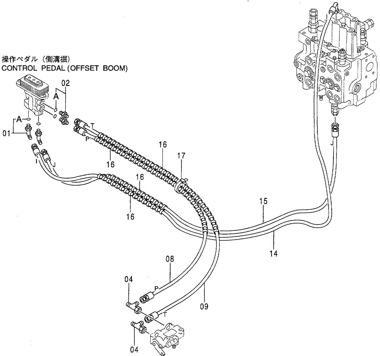
パイロット配管 (7) PILOT PIPING (7)
