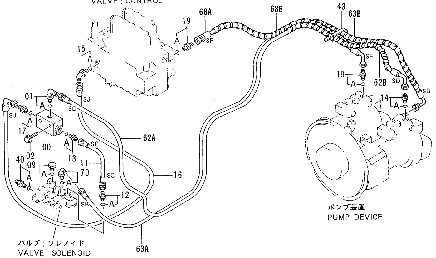
バルブ ; コントロール VALVE ; CONTROL
