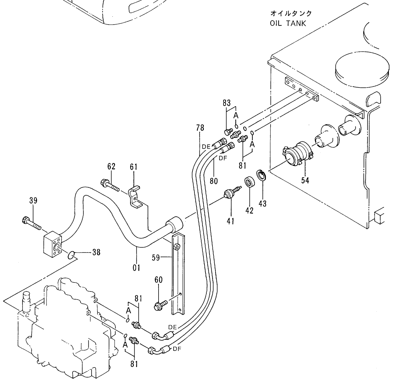
バルブ; コントロール VALVE; CONTROL
