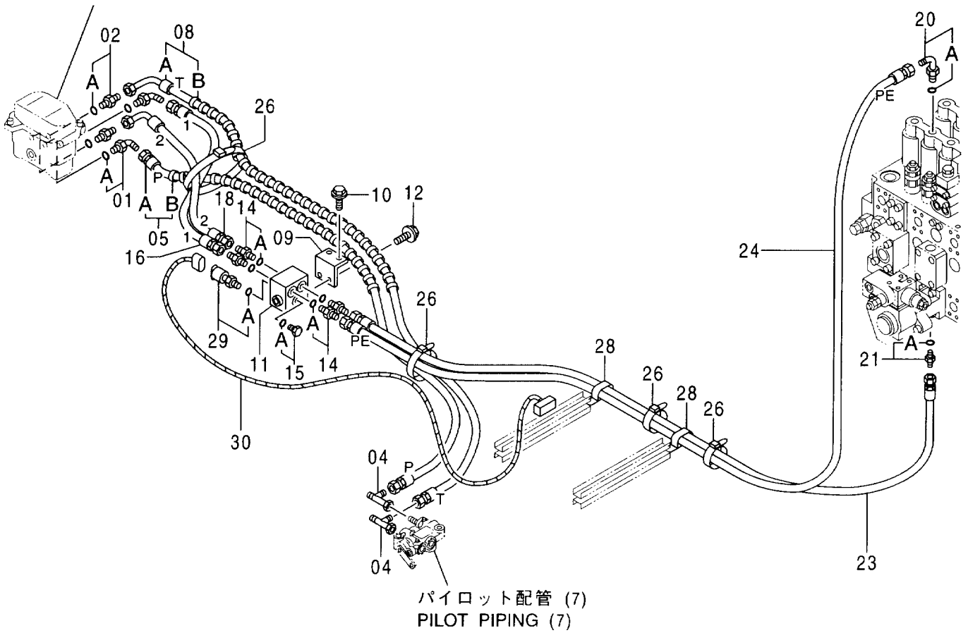
操作ペダル (ブレーカ & クラッシャ) CONTROL PEDAL (BREAKER & CRUSHER)
