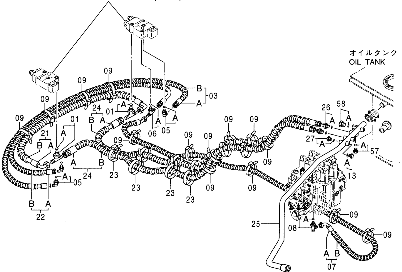
ホースラプチャバルブ配管 (ブーム) HOSE RUPTURE VALVE PIPING (BOOM)
