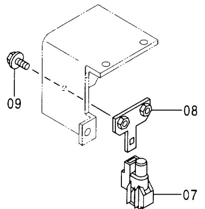
電気部品 (D) ELECTRIC PARTS (D)
