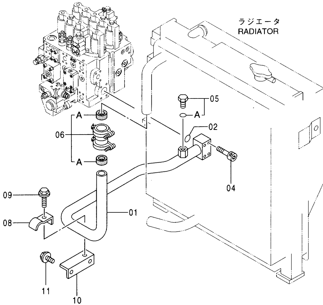
コントロールバルブ CONTROL VALVE
