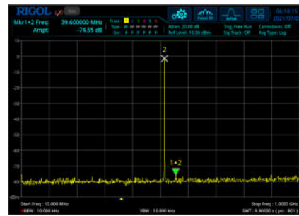
-70 dBc SFDR
