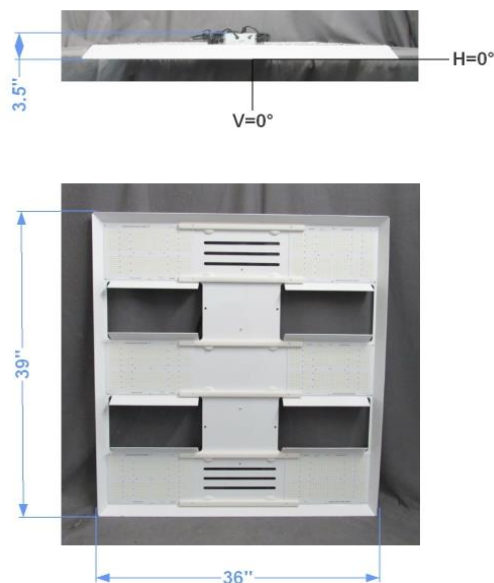
FIG. 1 LUMINAIRE
