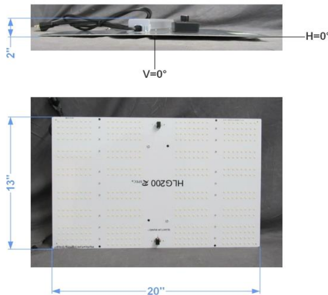
FIG. 1 LUMINAIRE
