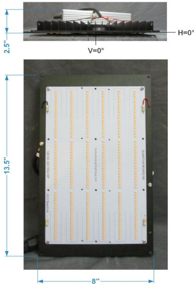
FIG. 1 LUMINAIRE
