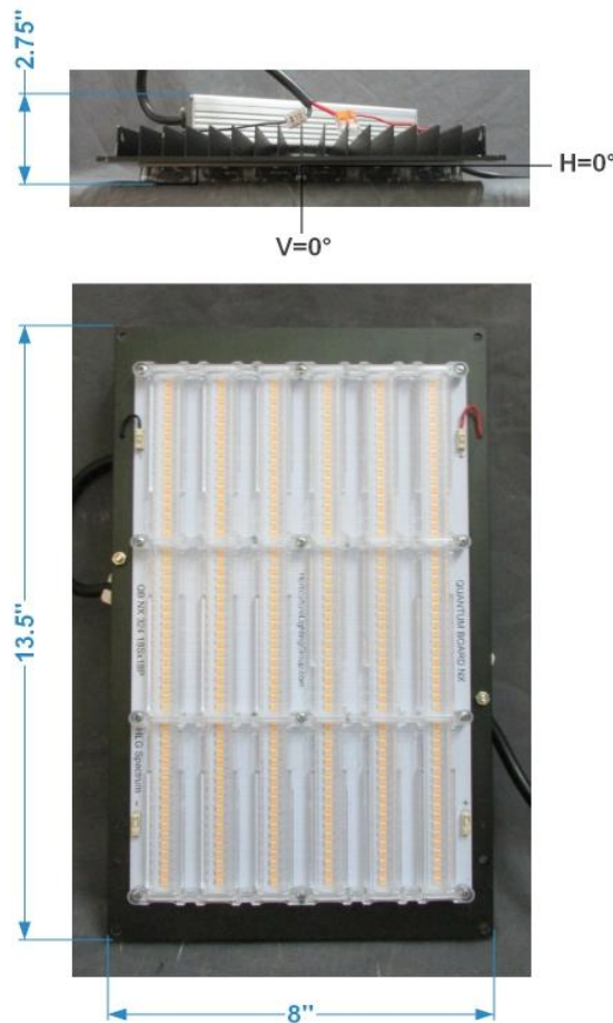
FIG. 1 LUMINAIRE
