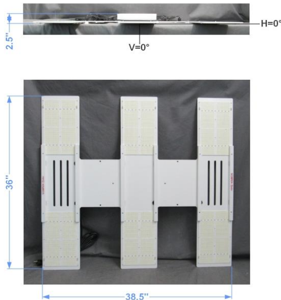
FIG. 1 LUMINAIRE
