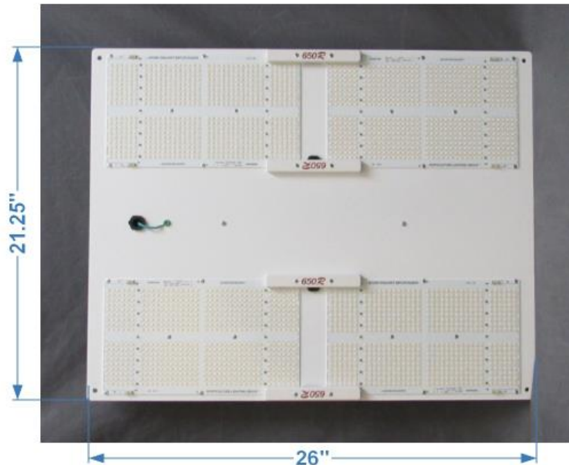
FIG. 1 LUMINAIRE
