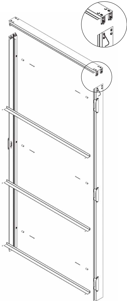
FRAME TYPE V - 45° FRAME
