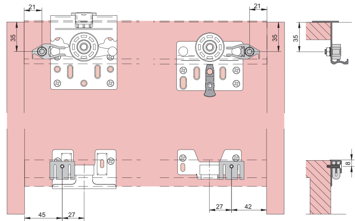
3 Instalação travões
