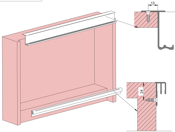
2 Montagem perfil
