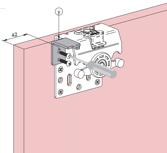
6a Instalação porta interior
