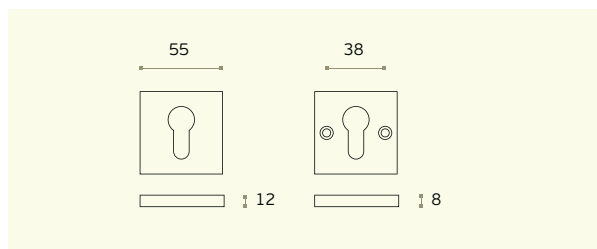
IN.04.36S Escudete de segurança para cilindro europeu / Security protection rose for european cylinder / Escudo de seguridad para bombillo. SÓLIDO / SOLID / MACIZO Material: EN 1.4301 - Satinado / Satin / Satin
