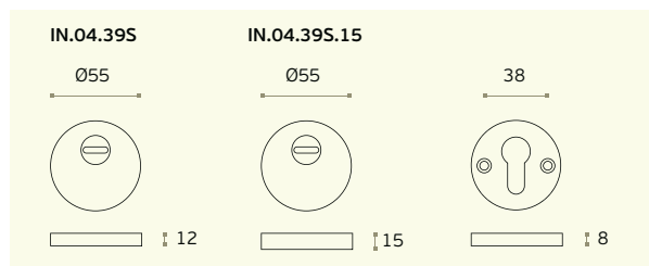
IN.04.39S / IN.04.39S.15 Escudete de segurança ajustável para cilindro europeu / Adjustable security protection rose for european cylinder / Escudo de seguridad ajustable para bombillo. SÓLIDO / SOLID / MACIZO Material: EN 1.4301 - Satinado / Satin / Satin
