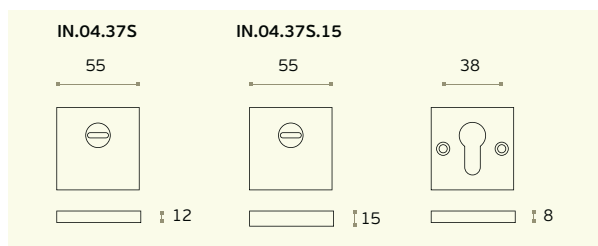
IN.04.37S / IN.04.37S.15 Escudete de segurança ajustável para cilindro europeu / Adjustable security protection rose for european cylinder / Escudo de seguridad ajustable para bombillo. SÓLIDO / SOLID / MACIZO Material: EN 1.4301 - Satinado / Satin / Satin
