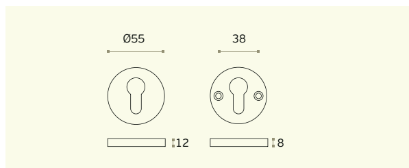
IN.04.38S Escudete de segurança para cilindro europeu / Security protection rose for european cylinder / Escudo de seguridad para bombillo. SÓLIDO / SOLID / MACIZO Material: EN 1.4301 - Satinado / Satin / Satin
