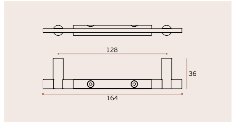
IN.22.280 Soft EN 1.4301-Satinado/Satin/Satin Asa de móvel/ Furniture handle / Tirador de mueble /
