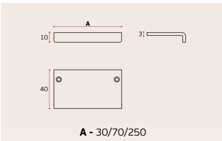
IN.22.119 EN 1.4301-Satinado/Satin/Satin Asa de móvel/ Furniture handle / Tirador de mueble.
