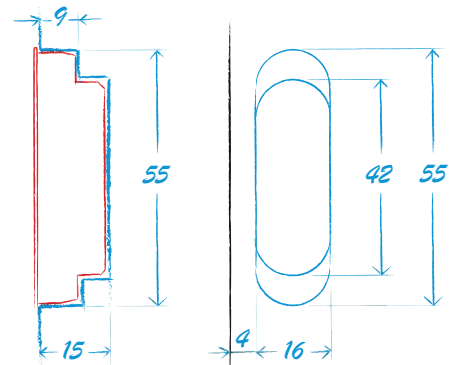
fresado en el marco para puerta solapada
