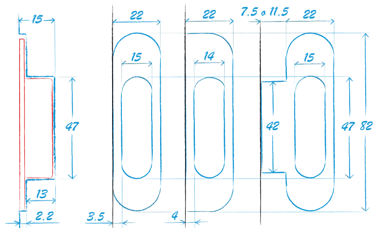
fresado en el marco para puerta solapada
