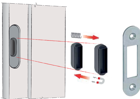
Ejemplo de fresado en el marco para puerta solapada
