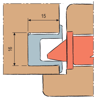
Aplicación en puertas solapadas con Mediana Evolution
