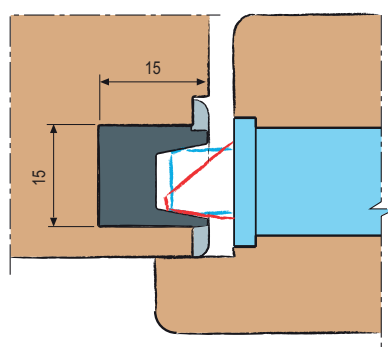
Aplicación Easy-matic en puertas solapadas con cerradura Mediana
