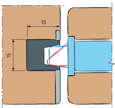
Aplicación Easy-matic en puertas lisas con cerradura Mediana
