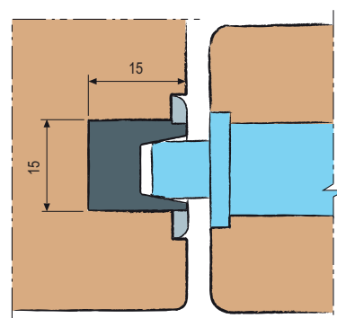
Aplicación en puertas lisas con cerradura Mediana Polaris
