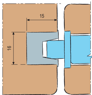
Aplicación en puertas lisas con Mediana Polaris
