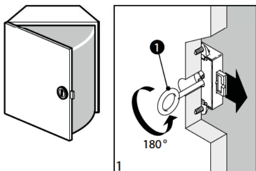
Bild 1 Bartschlüssel 1 um 180° gegen den Uhrzeigersinn drehen. Riegel wird rausgeschossen.
