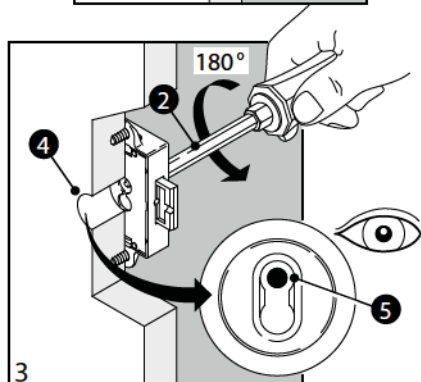
Bild 3 Kreuzschlitzschraubendreher 2 um 180° im Uhrzeigersinn drehen. Sichtkontrolle 4, Führungsbolzen 5 steht oben.
