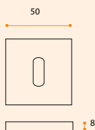
IN.04.29Q.P08.N QUADRO Material: EN 1.4301 - Satinado / Satin / Satin Entrada de chave normal / Key hole for normal key / Bocallave para llave normal.
