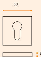
IN.04.29Q.Y08.N QUADRO Material: EN 1.4301 - Satinado / Satin / Satin Entrada para cilindro europeu / Key hole for european cylinder / Bocallave para bombillo europeu.
