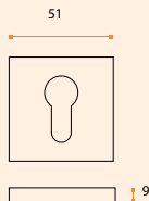
IN.04.29Q.Y09.M QUADRO IN.04.29Q.Y09.MP QUADRO Material: EN 1.4301 - Satinado / Satin / Satin Entrada para cilindro europeo / Key hole for european cylinder / Bocallave para bombillo europeo.
