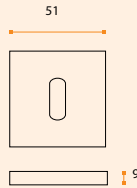
IN.04.29Q.P09.M QUADRO IN.04.29Q.P09.MP QUADRO Material: EN 1.4301 - Satinado / Satin / Satin Entrada de chave normal / Key hole for normal key / Bocallave para llave normal.
