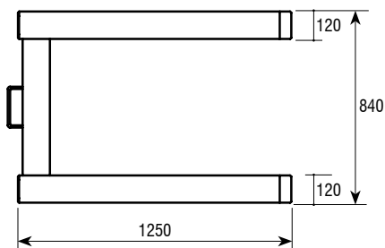
Dimensiones (mm)
