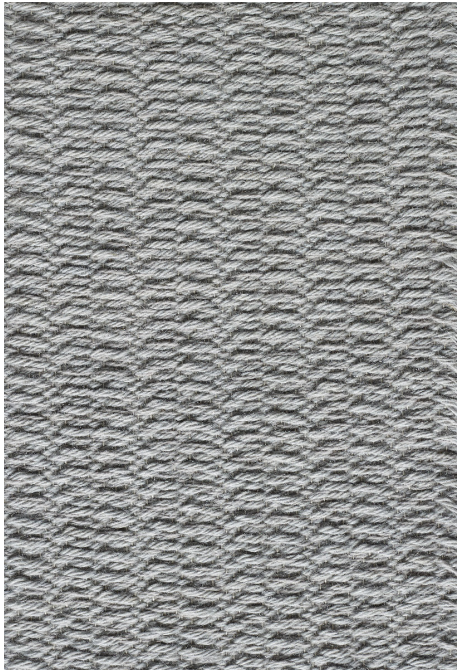
PUMICE
