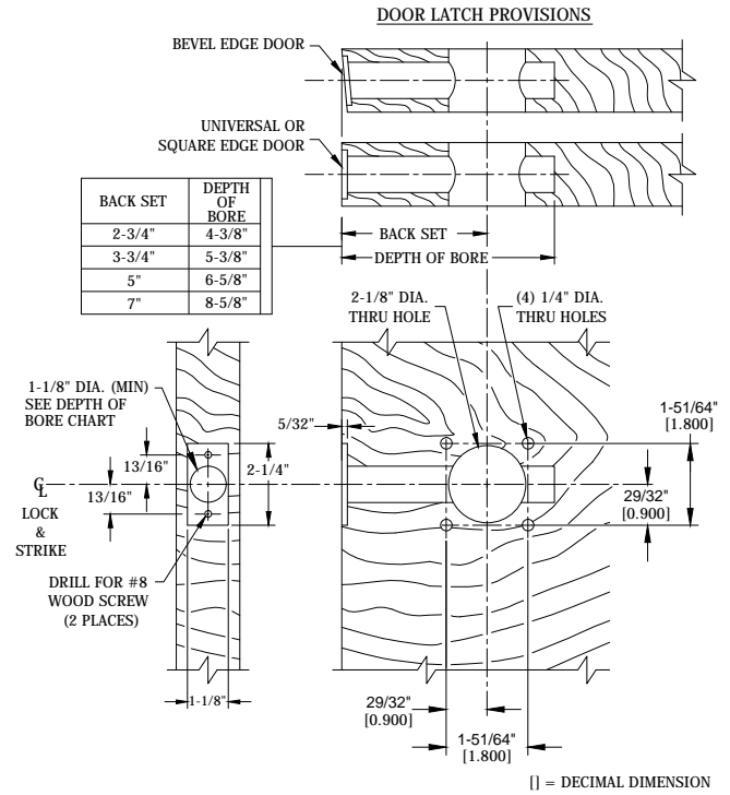
WOOD DOOR
