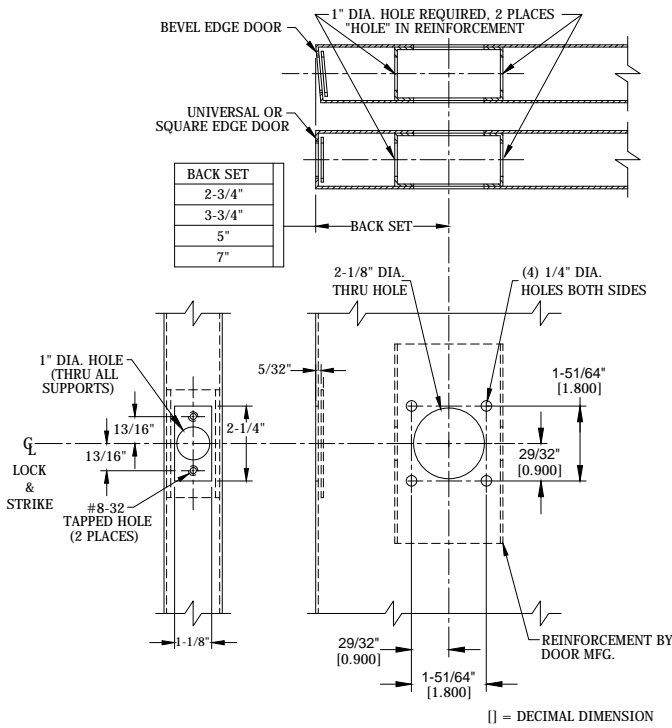
METAL DOOR
