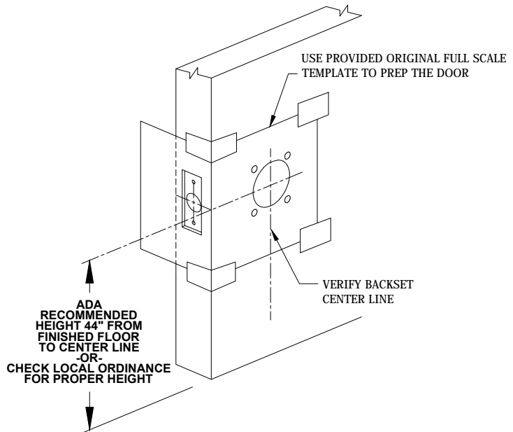
WOOD DOOR
