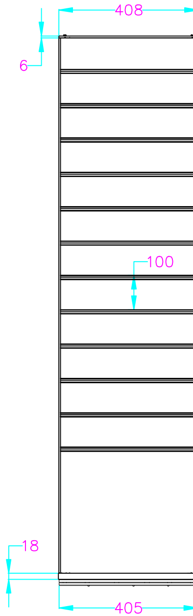
End elevation
