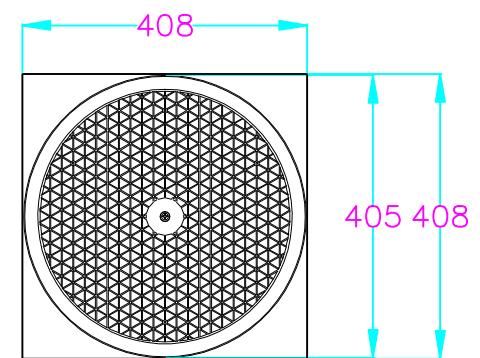
Bottom elevation
