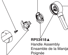
RP53417 ▲ Temperature Knob and Cover Perilla de la Temperatura y Cubierta Poignée de Réglage de Température
