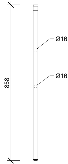
Seitenansicht side view
