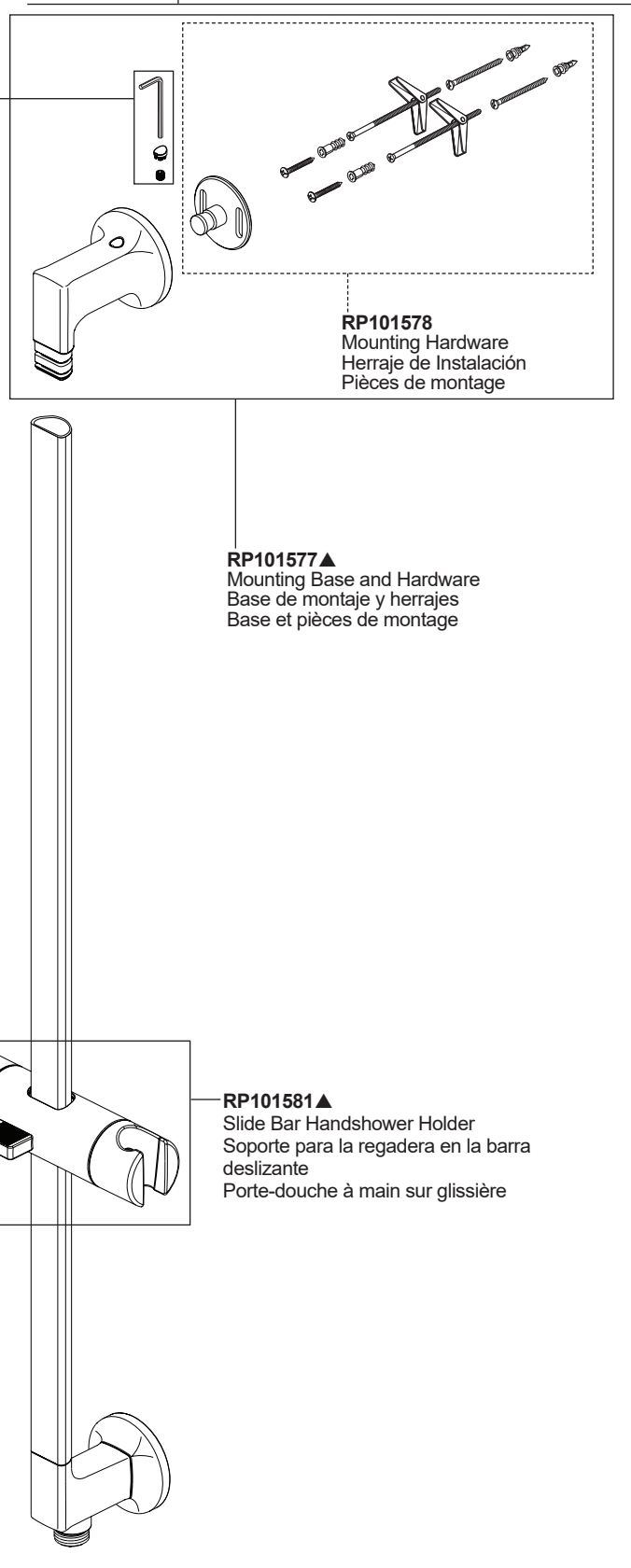
RP101580▲ Slide Bar Assembly Conjunto de la Barra Corrediza Coulisse avec ses éléments
