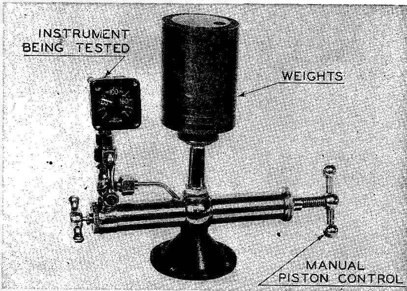
Ⓐ Low range.
