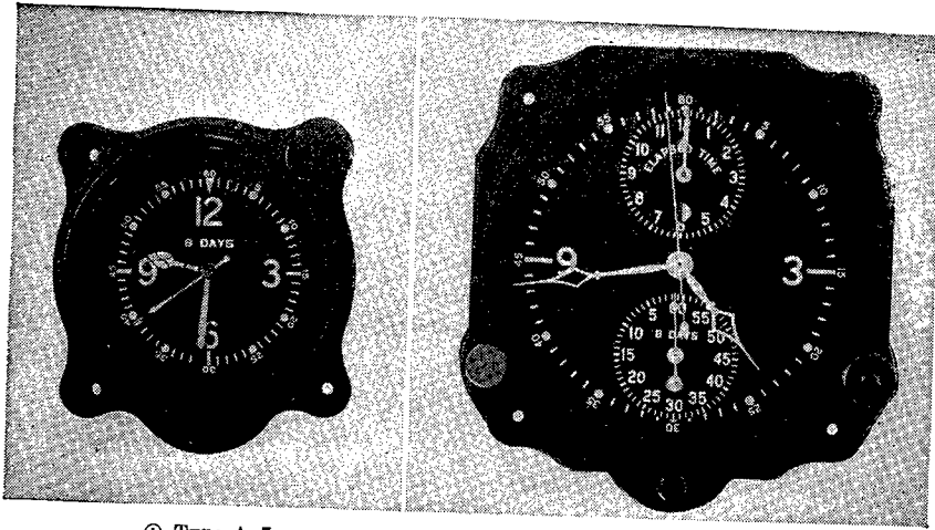
⊙ Type A-8.
