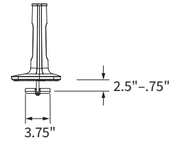
Grommet
