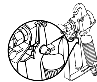
G-08/10 pistola cerrada (pistola no pintará)
