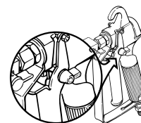
G-08/10 pistolet bloqué (le pistolet ne peut pas pulvériser)
