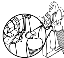
G-08/10 pistolet bloqué (le pistolet ne peut pas pulvériser)
