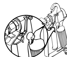
G-08/10 desbloqueada (La pistola pulveriza)
