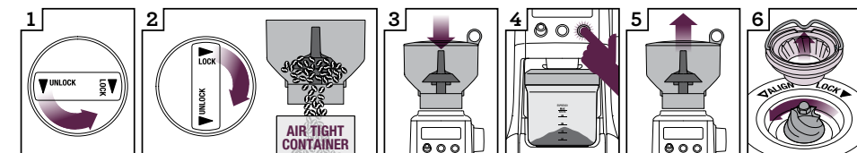
1 Déverrouillez la trémie 2 Tenez la trémie au-dessus du contenant pour distribuer les grains 3 Alignez la trémie 4 Faites fonctionner pour vider 5 Retirez la trémie 6 Retirez la meule supérieure
