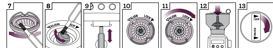
7 Nettoyez la meule supérieure avec la brosse 8 Nettoyez la meule inférieure avec la brosse 9 Nettoyez la sortie de mouture avec la brosse 10 Enfoncez la meule supérieure en place 11 Verrouillez la meule supérieure 12 Alignez la trémie en place 13 Verrouillez la trémie
