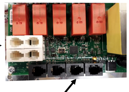
Figure 5 . Ordre des connecteurs RJ 10. Capteur, interrupteur de porte, télécommande, capteur NTC supplémentaire.
