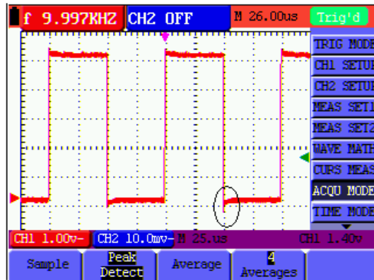
Abbildung 15: Spitzen-Messung
