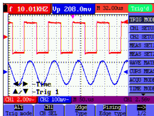
Abbildung 43: Alternate Trigger
