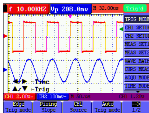
Abbildung 38: Flanken-Triggen
