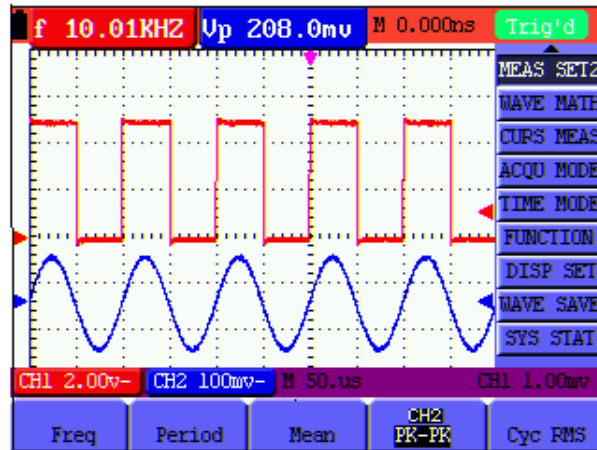
Abbildung 11: automatische Oszilloskop-Messungen
