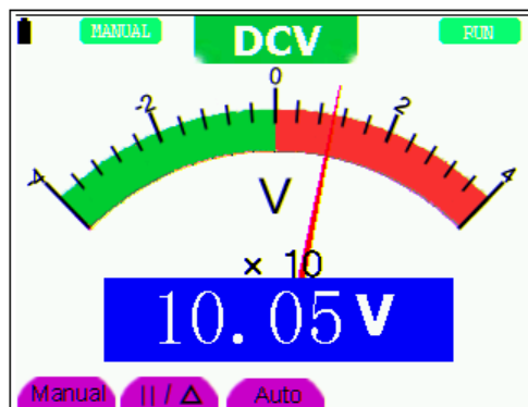
Abbildung 33: automatischen/manuellen Bereichswahl
