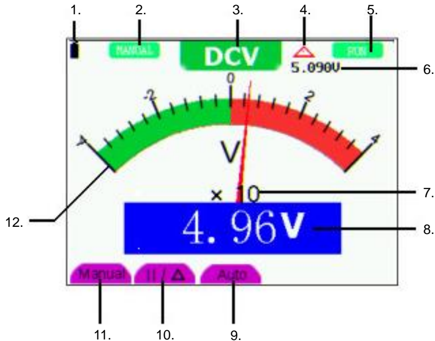
Abbildung 20: Betriebsanzeige DMM
