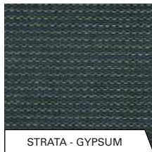
STRATA - GYPSUM
