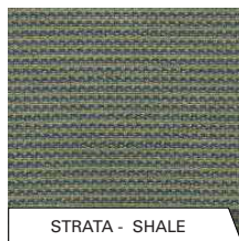
STRATA - SHALE
