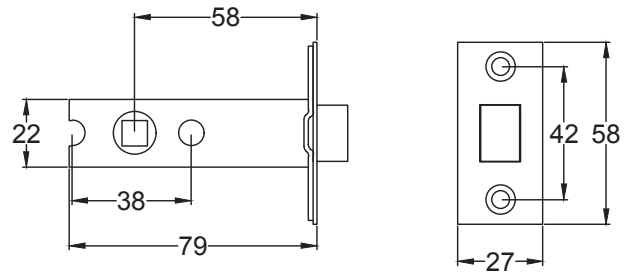
Tubular Latch
