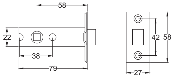
Tubular Latch
