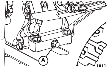
Figure 4-7. Bouchon de vidange de l'huile
