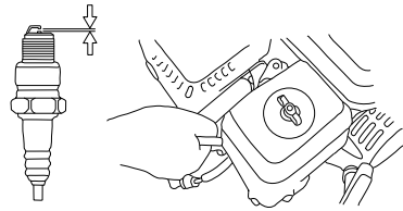
Figura 4-8. Bujía
