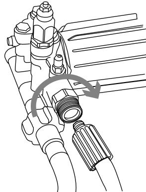
Figure 2-11. Raccord du tuyau à haute pression à la pompe
