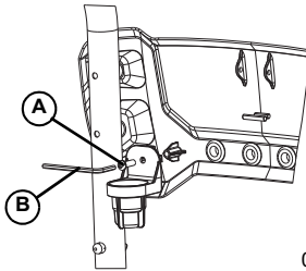
Figura 2-3. Soporte de la boquilla/accesorios
