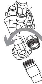
Figura 2-11. Conexión de la manguera del suministro de agua
