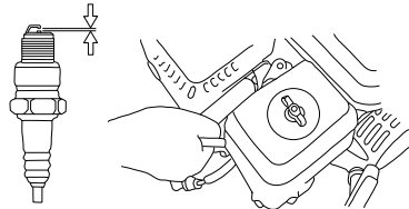
Figure 4-8. Bougie d'allumage
