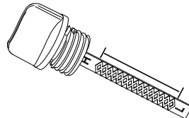
Figure 2-8. Plage de fonctionnement sûr
