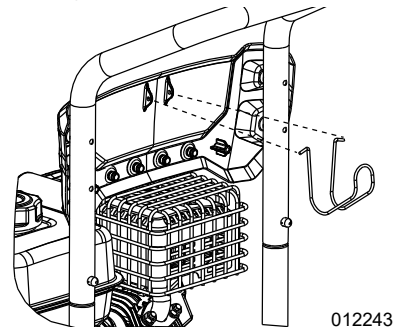
Figura 2-2. Instalación del gancho de la manguera
