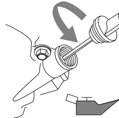
Figura 2-7. Extracción de la varilla
