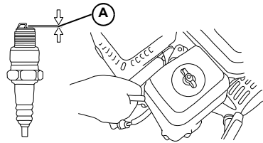
Figura 4-8. Bujía
