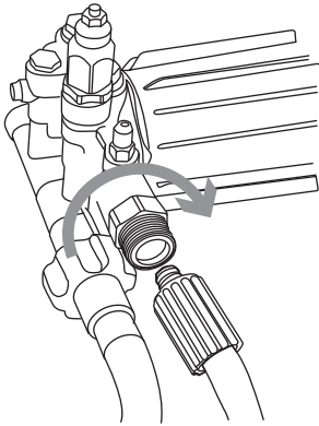
Figura 2-13. Conexión de la manguera de alta presión a la bomba
