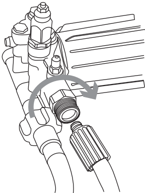
Figure 2-13. Raccordement du tuyau à haute pression à la pompe
