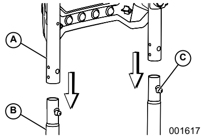
Figura 2-1. Inserción del asa
