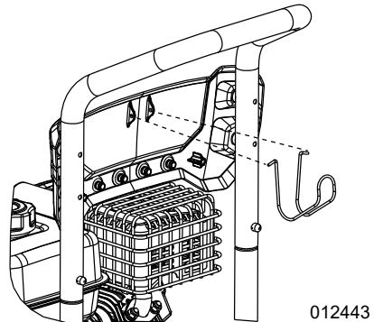
Figure 2-2. Installation du crochet du tuyau
