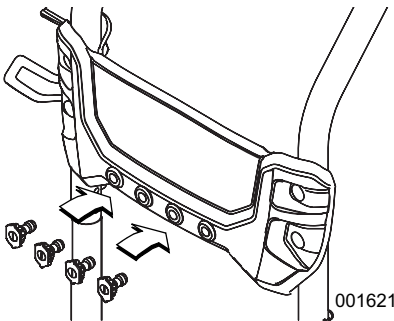
Figura 2-5. Inserción de las boquillas
