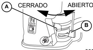
Figura 3-2. Válvula de combustible y cebador
