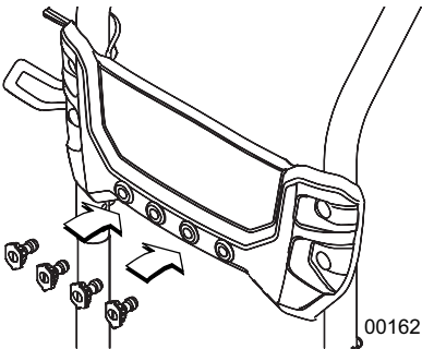
Figura 2-5. Inserción de las boquillas
