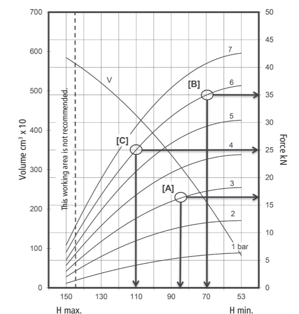
M-40 rubber bellow data chart Datendiagramm M-40 Balgzylinder
