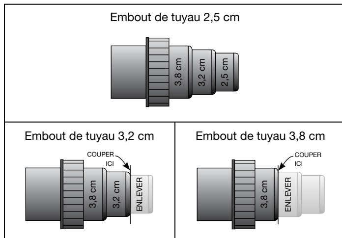
UltraKlear MD avec raccords à balle tournante et adaptateurs multi-tuyaux
