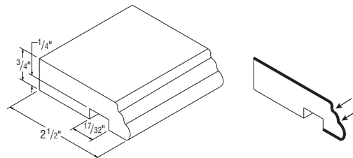
MTST8 (1 - 8' pc) PSMTST8 (1 - 8' pc)
