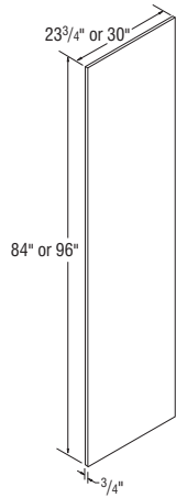
PREF2384 PREF2396 PREF3084 New PREF3096 New
