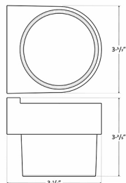
3 1/8"(W) x 3 2/5"(H) x 3 5/7"(D)
