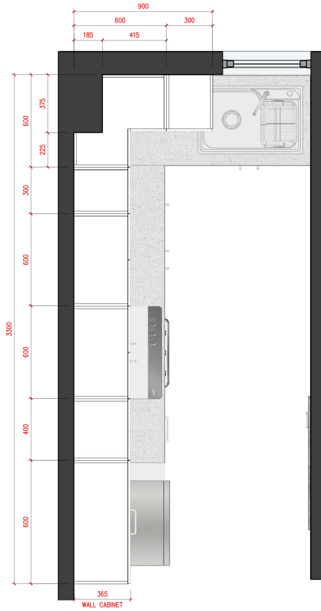
2 VNARES - TYPE 2B WALL CABINET LAYOUT SCALE: A3 A:15 MM
