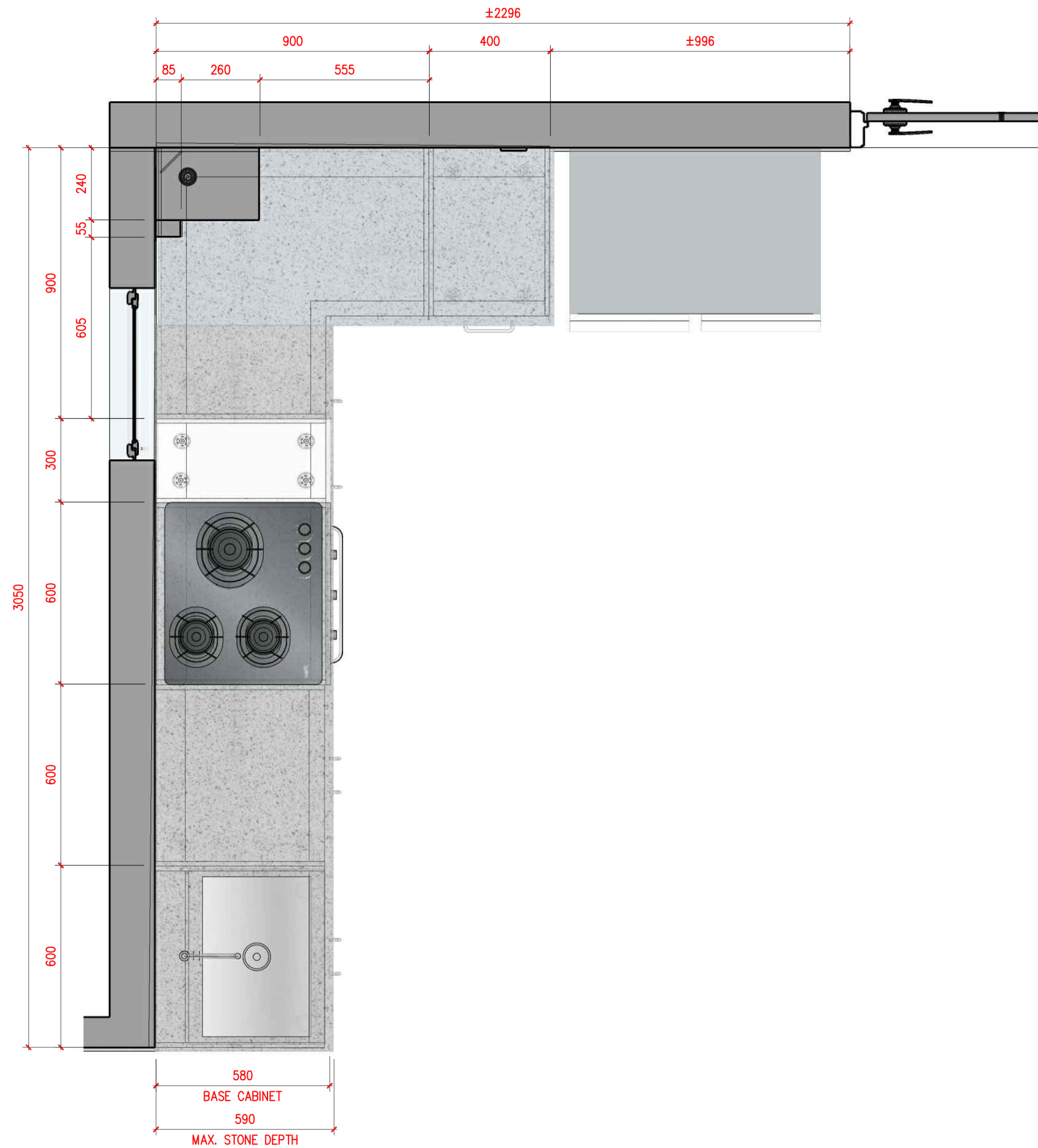
1 VNARES - TYPE 1C BASE CABINET LAYOUT SCALE: A3 A:15 MM
