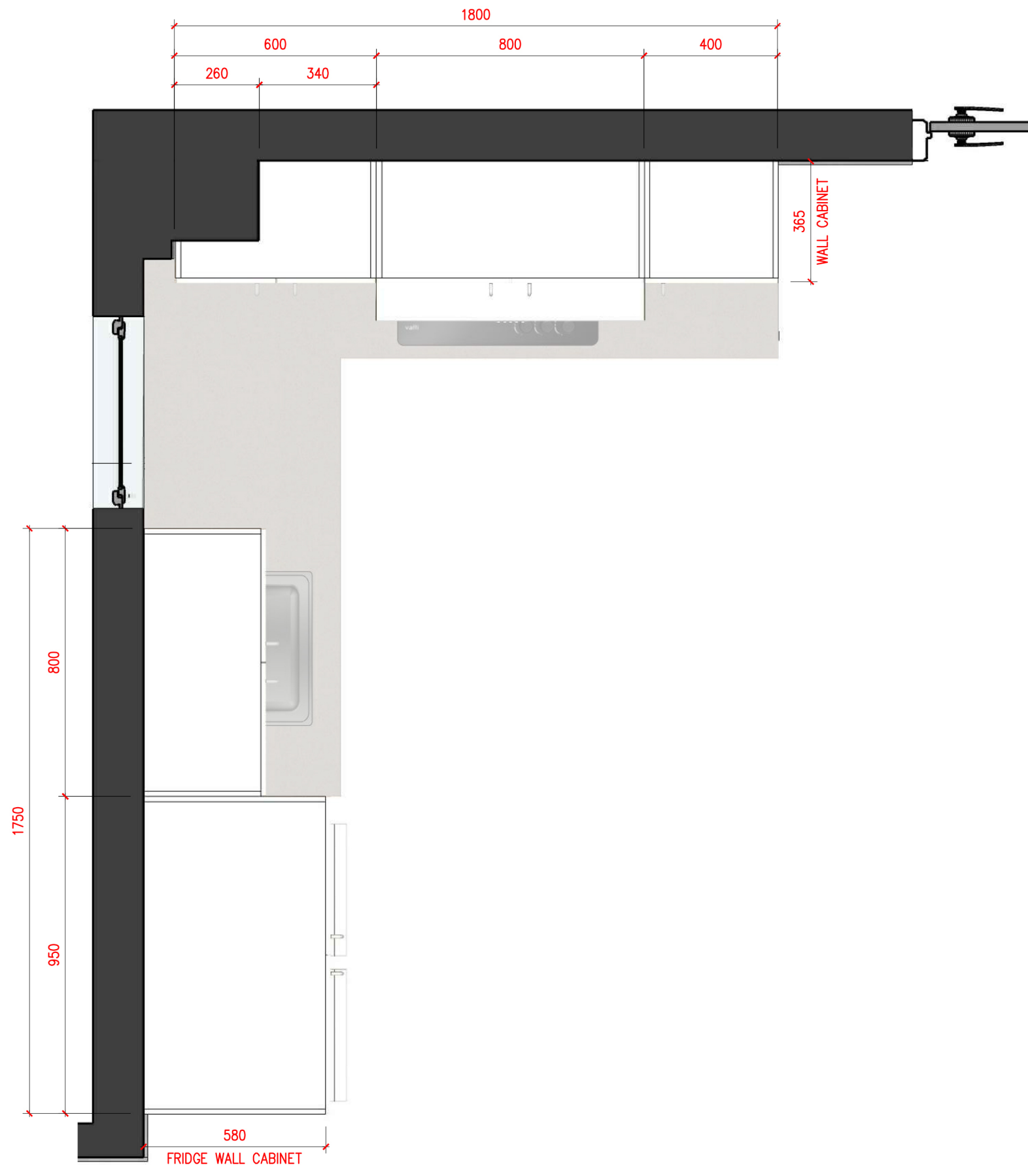
1 VNARES - TYPE 1A WALL CABINET LAYOUT SCALE: A3 A:15 MM
