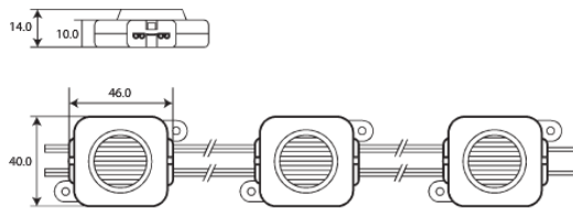
Z1U-V05(Edge Module)
